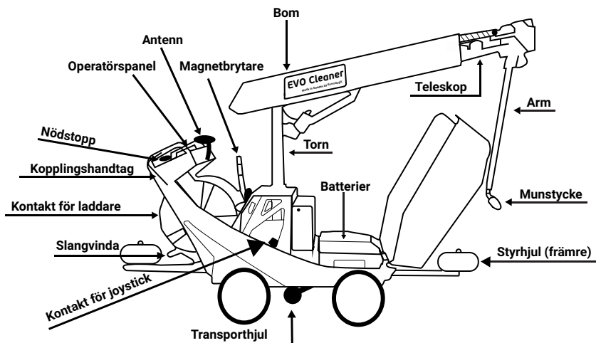
Figur 2, robotens delar
