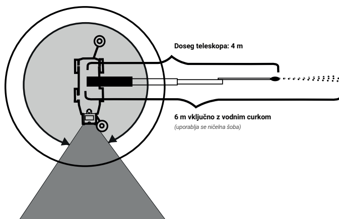
Slika 3, doseg manipulatorja in varno območje delovanja stolpa
