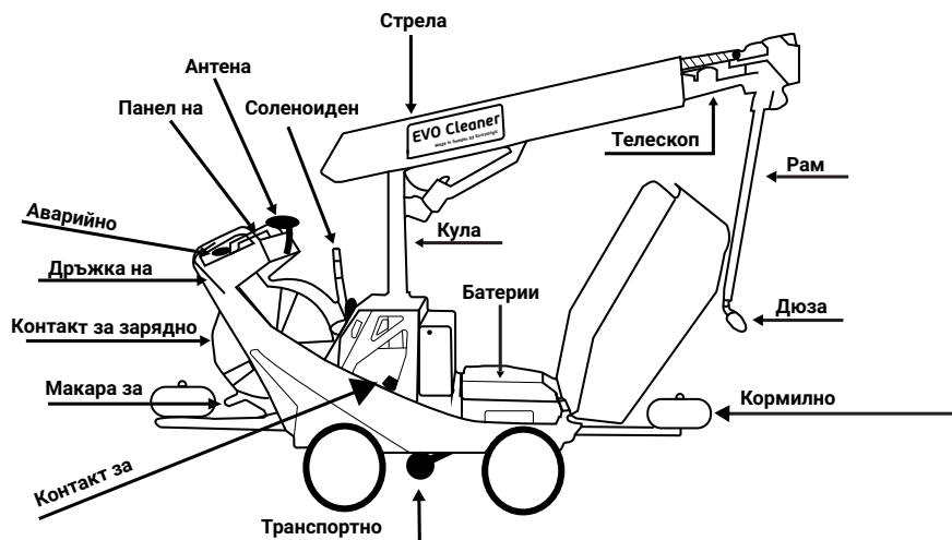
Фигура 2, части на робота
