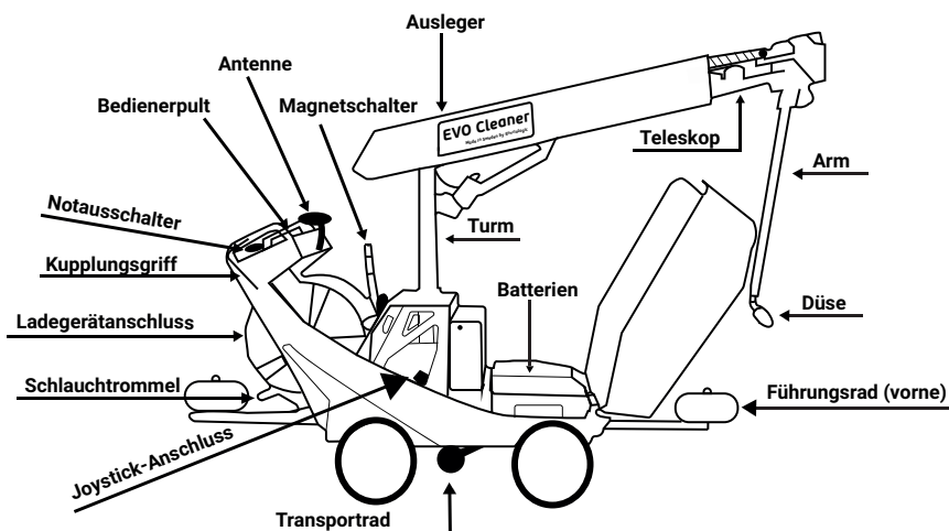
Abbildung 2, Teile des Roboters
