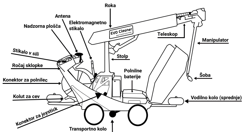
Slika 2, deli robota
