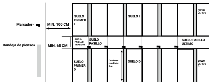
Figura 6, ejemplo de diseño de un corral de cerdos
