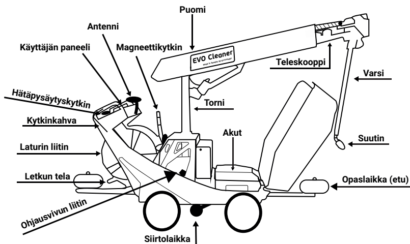
Kuva 2, robotin osat
